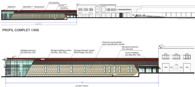
EXTRAIT SUR BATIMENT PROJETE 1/250
