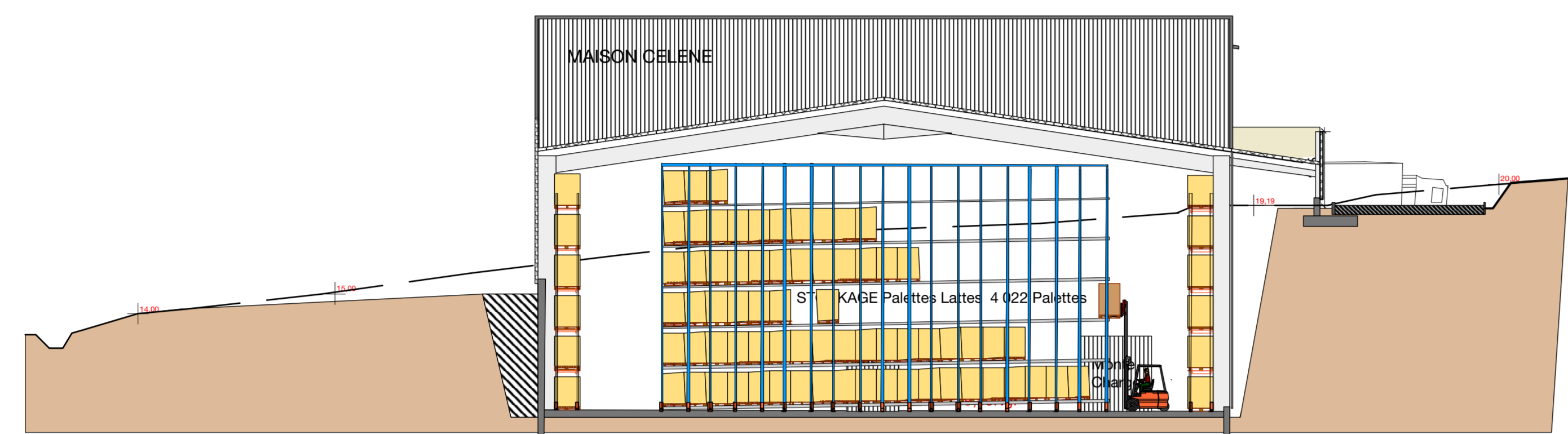
Coupe E-E
