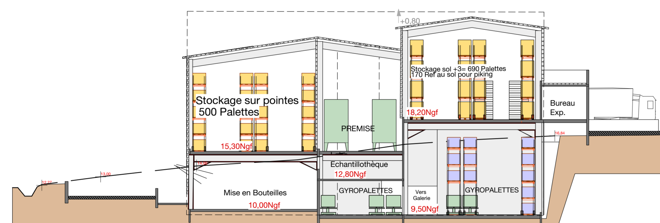
Coupe C-C
