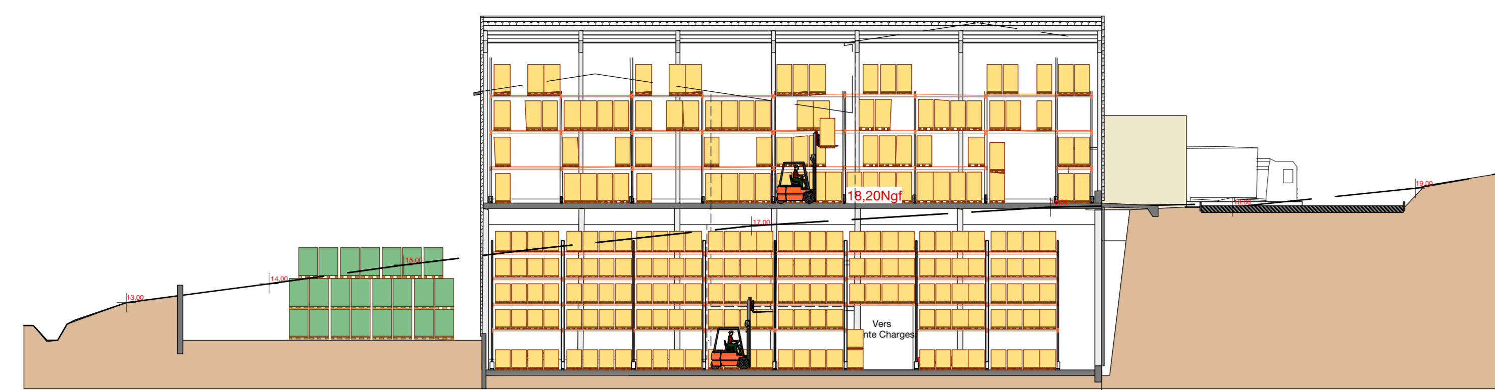
Coupe D-D
