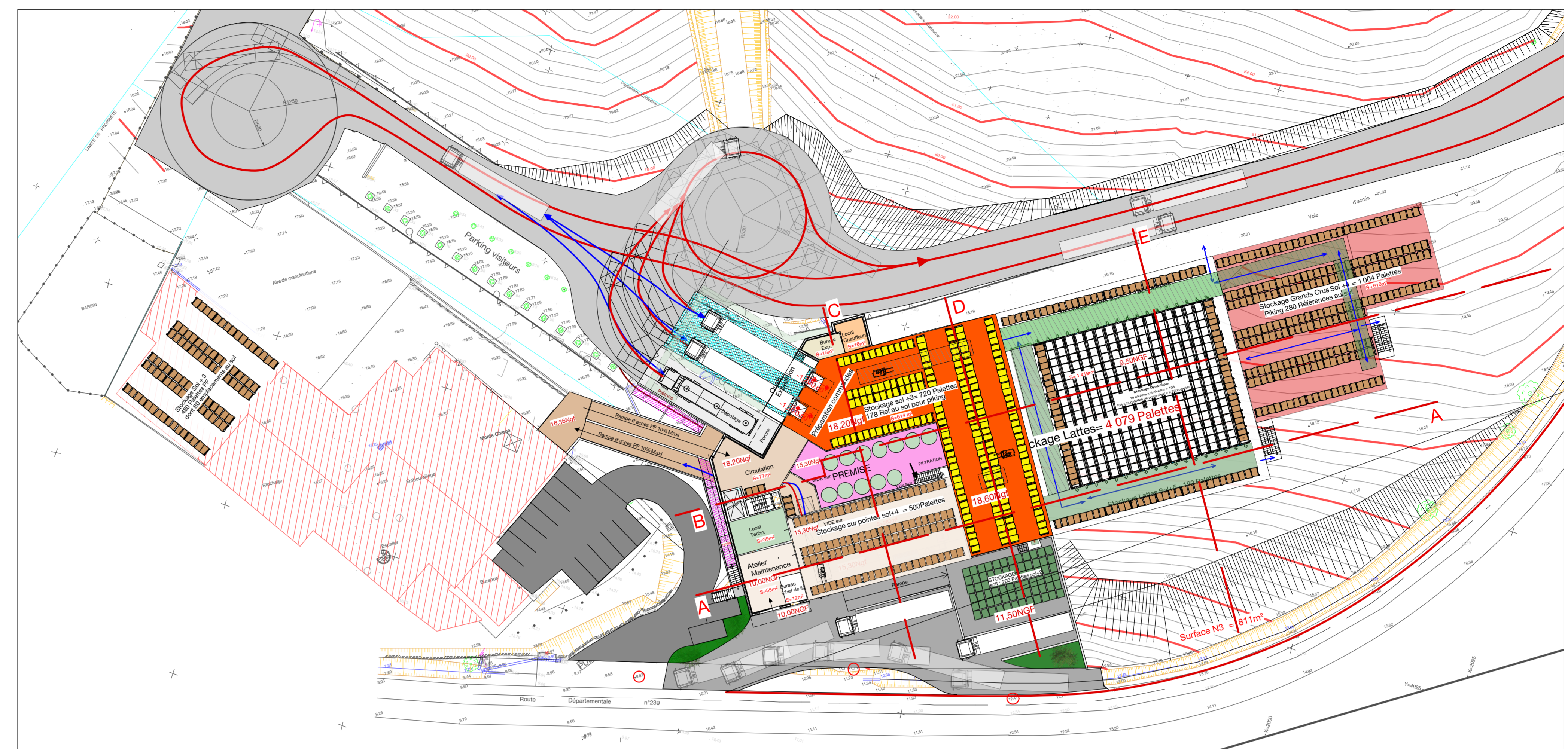
Repérage Ech: 1/400
